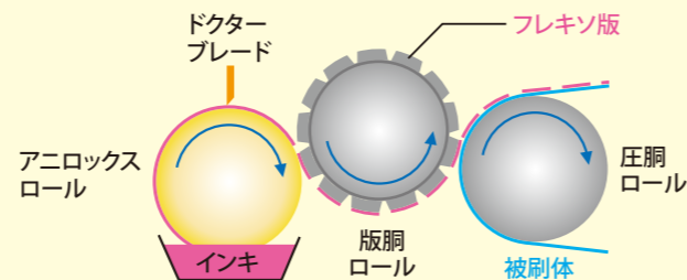
《フレキソ印刷のしくみ》
